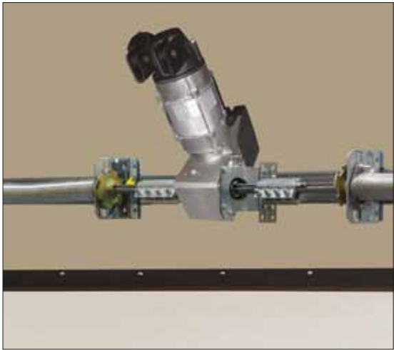
Крепление электропривода по центру
