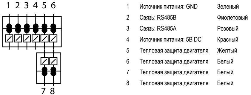
Рис. 9 Распайка клеммной колодки
