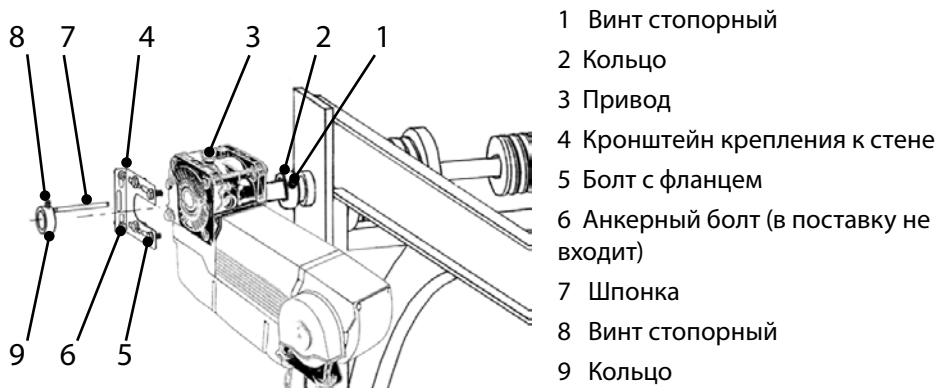
Рис.3 Схема установки привода на вал секционных ворот
